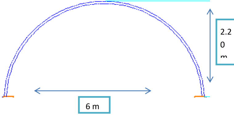
Şekil 1: ¾ inç çapında 2 mm et kalınlığında 8 m boyunda galvanizli su borusunun 6 m genişlik ve 2.2 m yükseklikte bükülmesi
