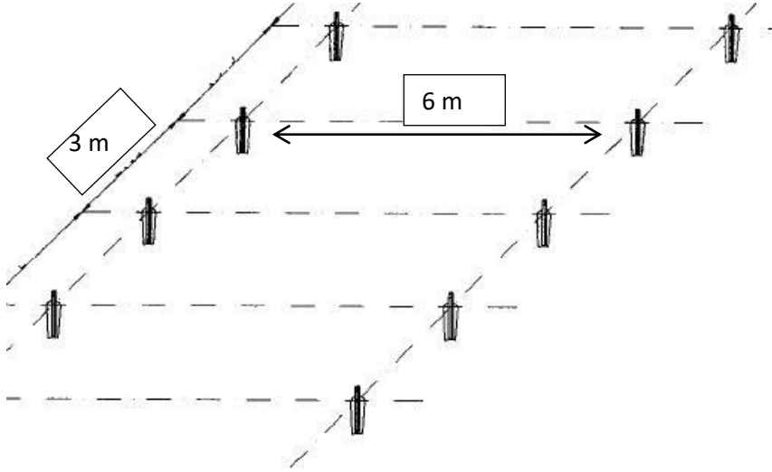
Şekil 3: Montaj için sabitleme demirlerinin yerleştirilmesi
